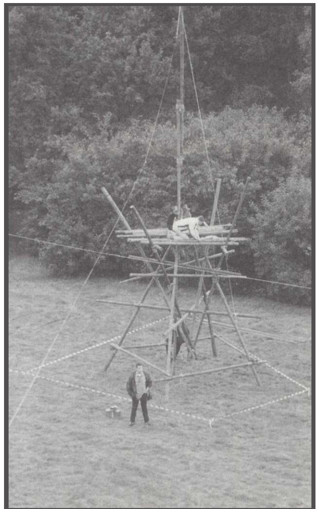
Antennemast
