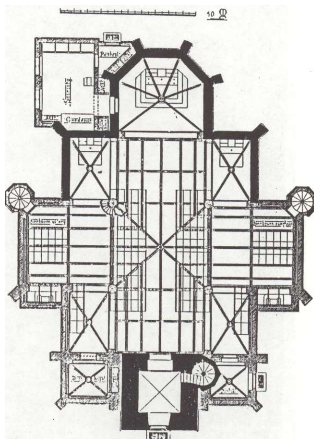
Plan tot herstel en vergroting van de kerk.
