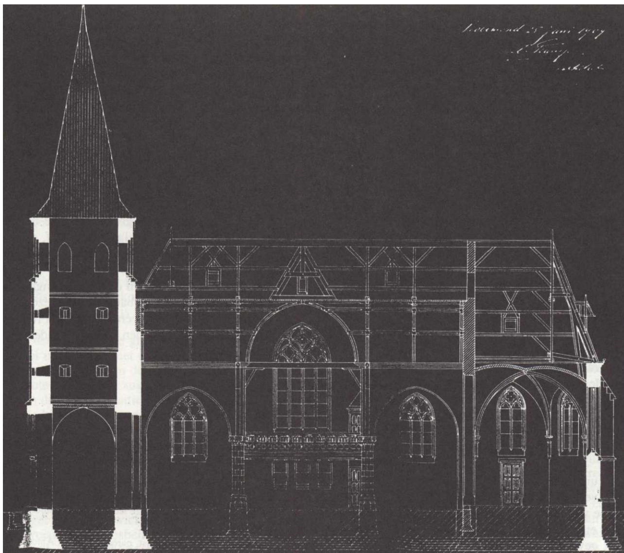
Werktekening van architect Franssen uit Roermond, met doorsnee van de aanbouw en kapconstructie.
