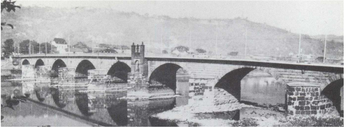
De Romeinse brug bij Trier. De bovenbouw is van latere datum, de pijlers zijn origineel. Waarschijnlijk is de pijlerconstructie van de brug tussen Middelaar en Cuijk een soortgelijke geweest.
